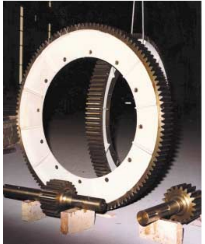
ENGRANAJE RECTO
