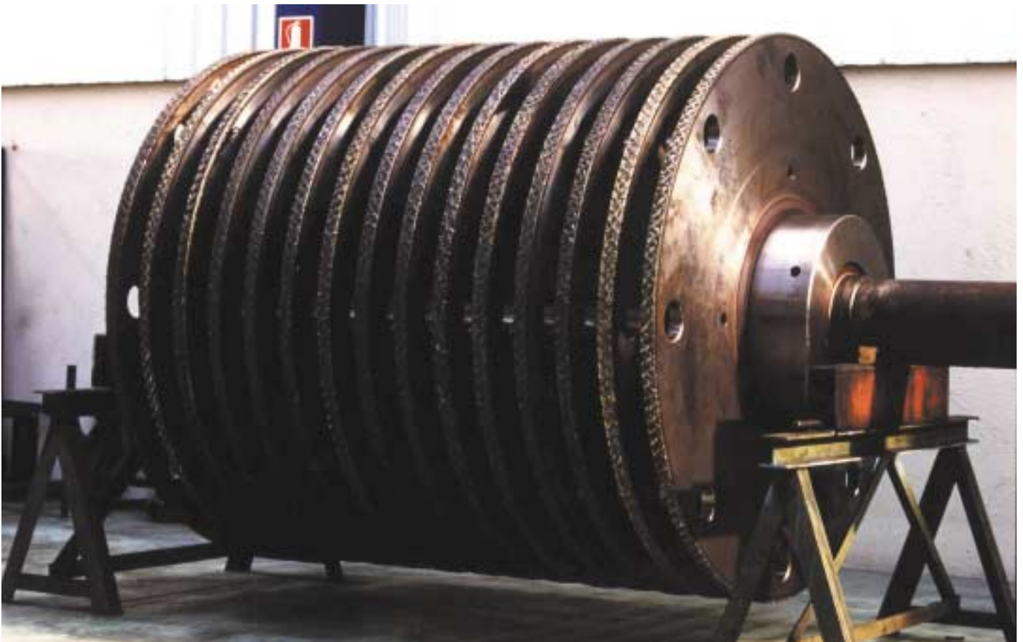
ROTOR DE CEMENTERA 32.000 KG.
