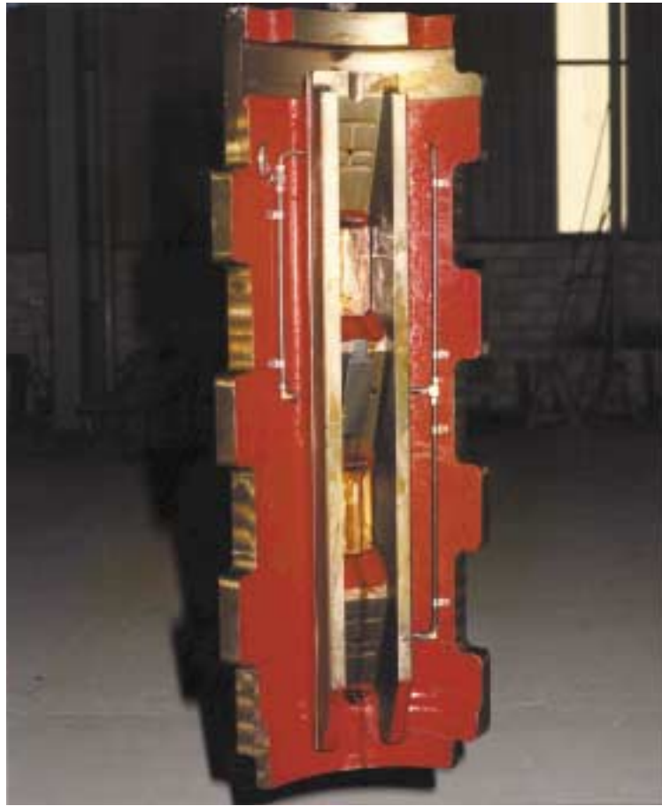
SEGMENTO EXPANSIONADOR. FUNDIDO PARA BOBINAS.
