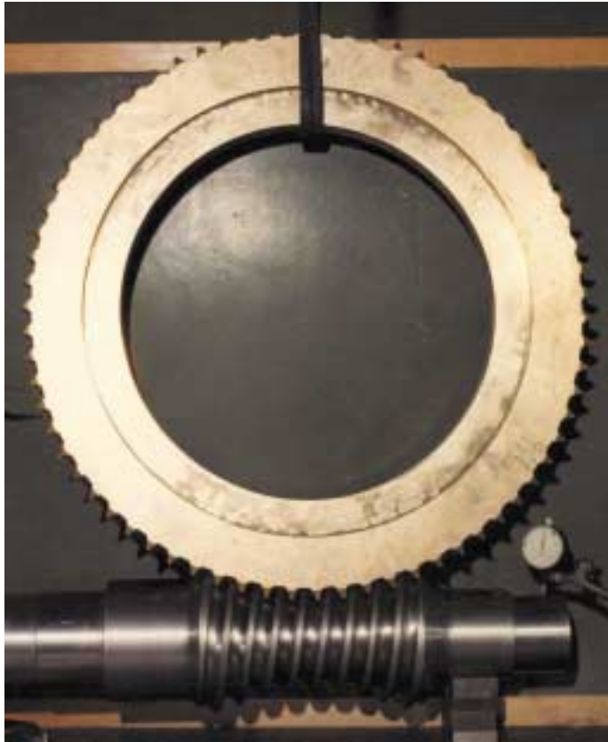
CORONA Y SINFIN GLOBOIDE DE 2 ENTRADAS
